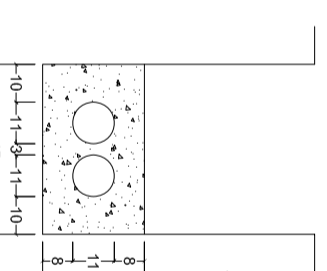
CANALIZACION EN ZANJA DE 2c. PVC. DE 110mm.
