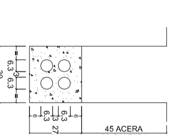
CANALIZACION EN ZANJA DE 4c. PVC. DE 63mm.
