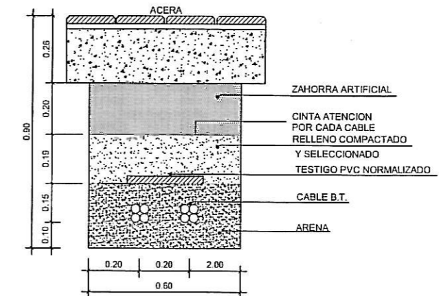
ZANJA PARA ANILLO DE BAJA TENSION BAJO ACERA Escala 1:200
