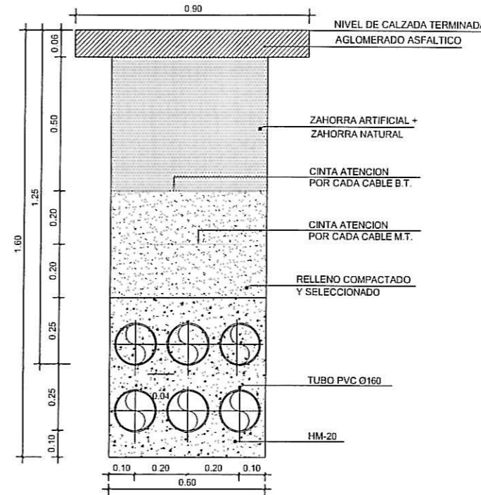
ZANJA B.T. CON UN ANILLO Y M.T. (TENDIDO DE CABLES EN CRUCES) Y BAJO CALZADA Escala 1:200
